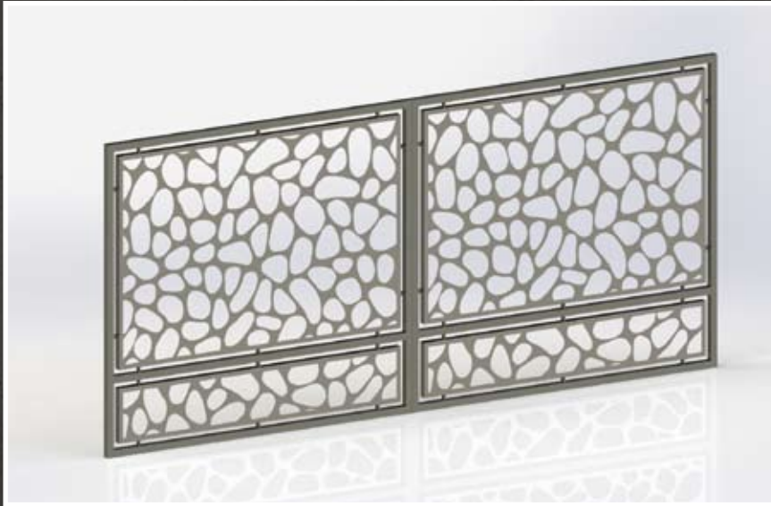
Brama skrzydłowa typu BS 01 szer. 390 cm (światło bramy 400 cm) wys. 150/160/170 cm
